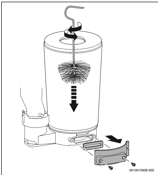
Obr. 59 Čištění tepelného výměníku
