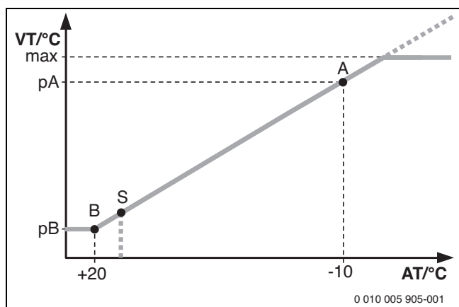
Obr. 84 Ekvitermní křivka
