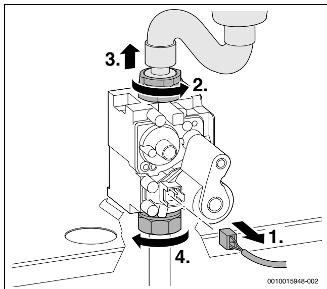
Obr. 71 Odpojení konektoru a povelení převlečných matic
