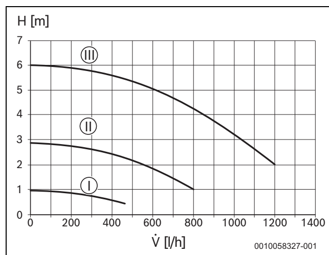
Obr. 45 Křivka čerpadla otopného systému (konstantní tlak)
