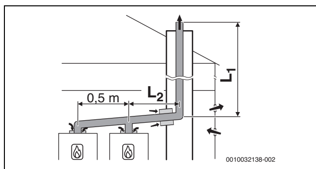
Obr. 28 Kaskáda se 2 zařízeními: Pevné vedení odtahu spalin v šachtě podle B 53p s přívodem vzduchu závislým na vzduchu z prostoru na zařízení
