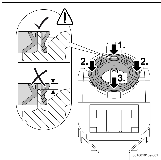
Obr. 66 Přitlačení těsnění
