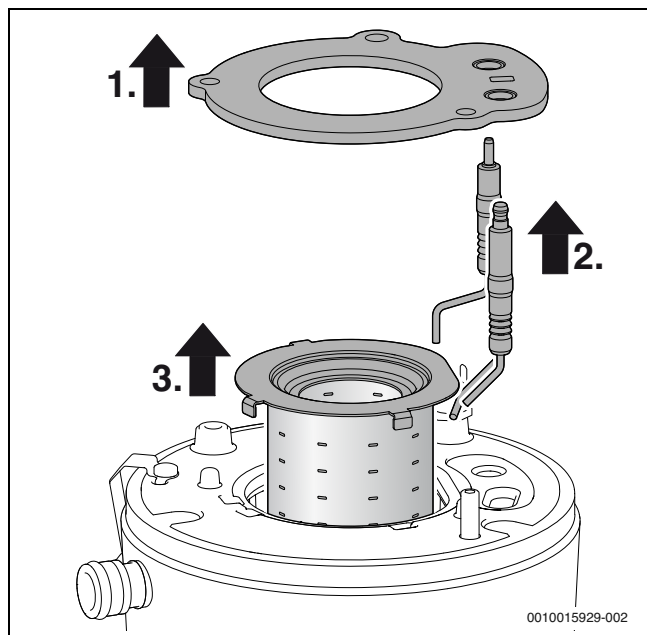
Obr. 56 Vyjmutí hořáku
