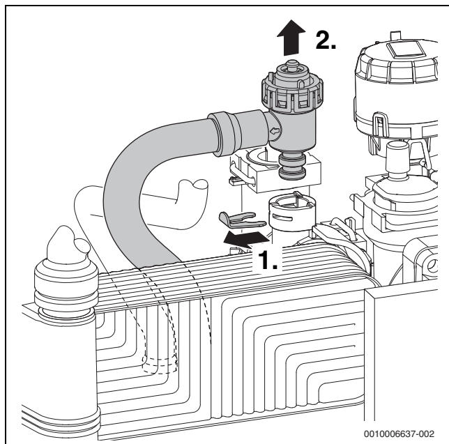
Obr. 68 Odebrání pojistného ventilu (otopný okruh)
