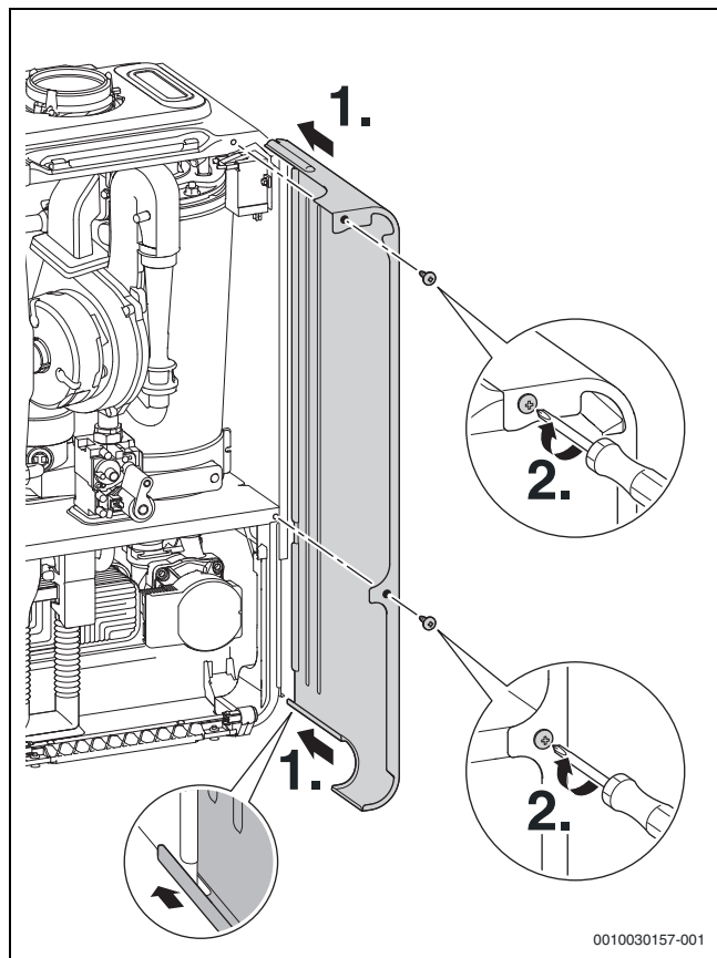
Obr. 80 Upevnění bočního opláštění
