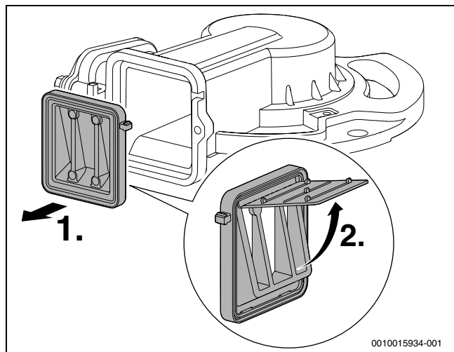
Obr. 55 Zpětná klapka ve směšovacím zařízení
