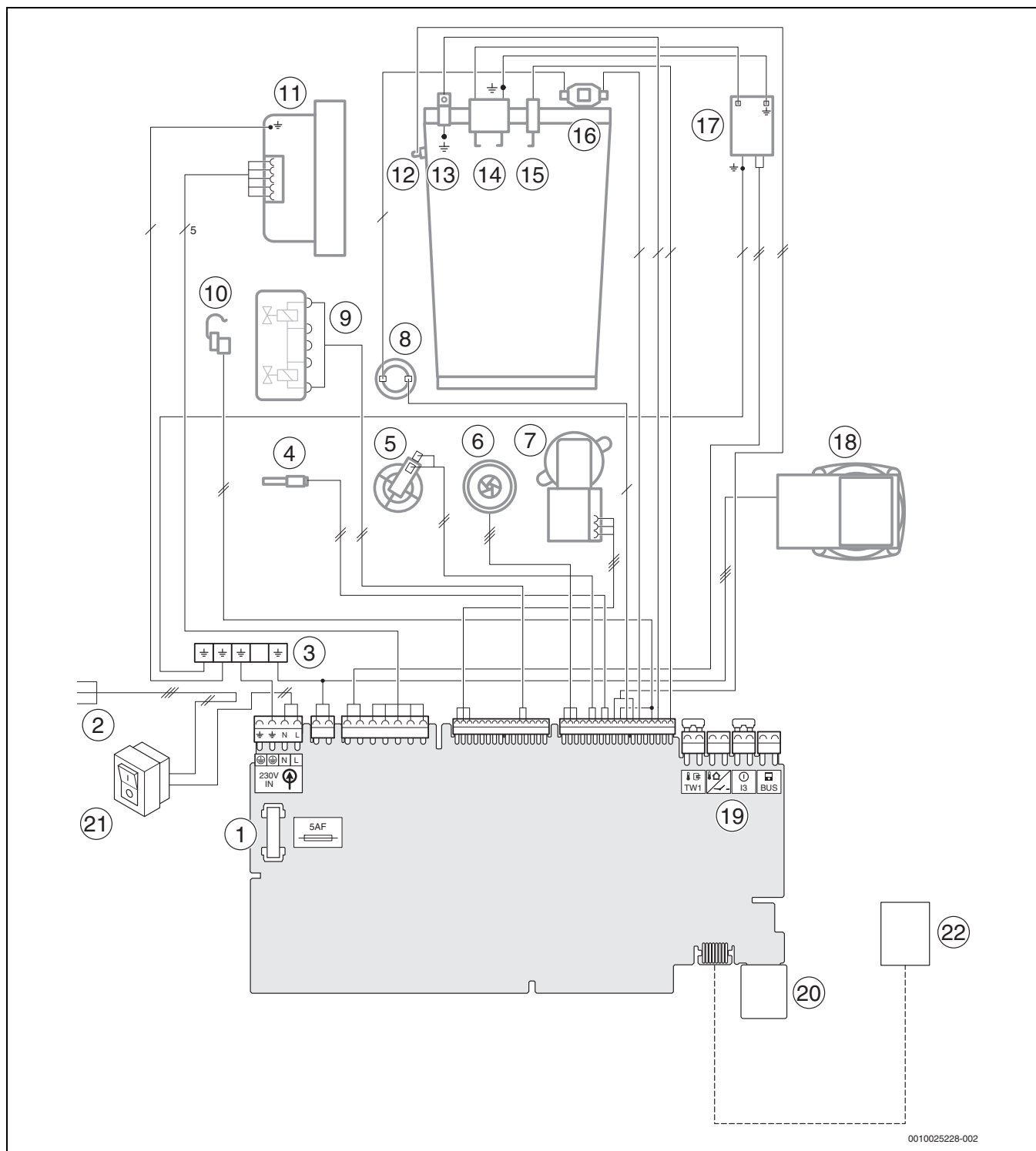
Obr. 83 Elektrické kabelové propojení
