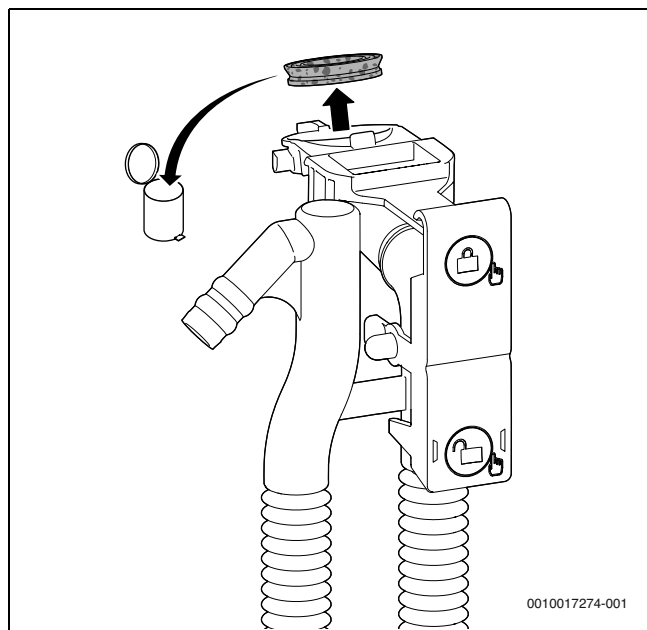
Obr. 64 Odstranění těsnění nahoře na sifonu kondenzátu
