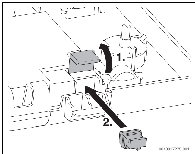
Obr. 79 Zasunutí kódovacího konektoru
