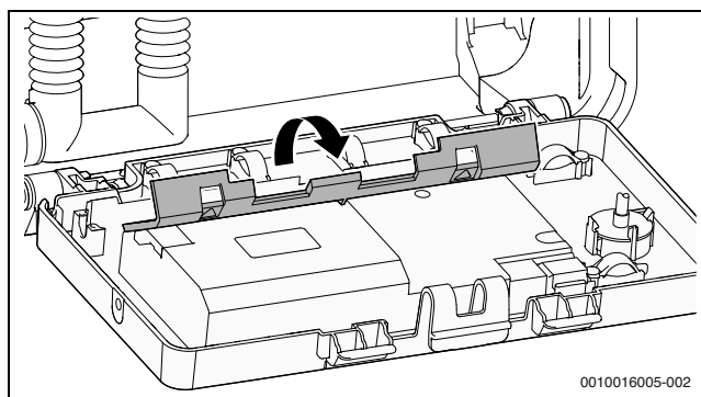
Obr. 39 Odklopení krytu
